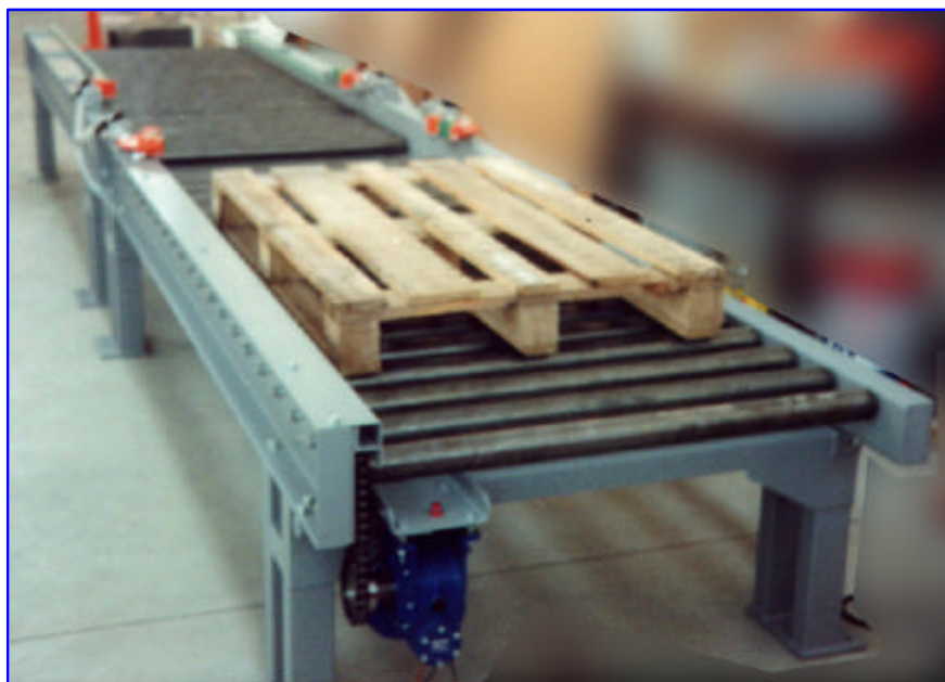
Foto 3.3 – Transportador a rodillos motorizados que lleva paletas
