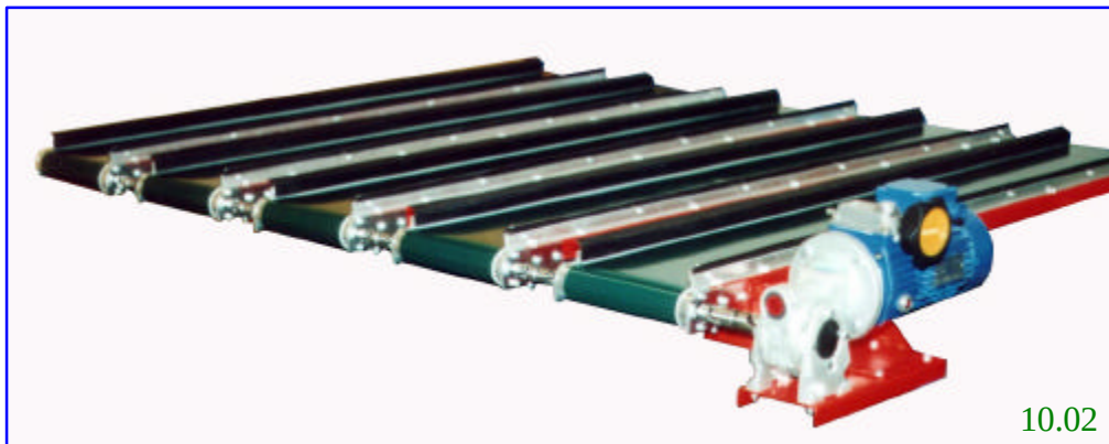
Transportadores juntados con transmisión movimiento a junta de Cardan
