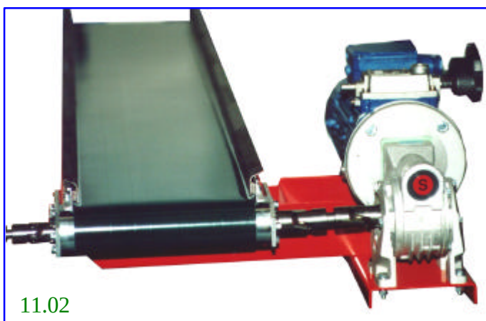
Transportadores juntados con transmisión movimiento a junta de Cardan
