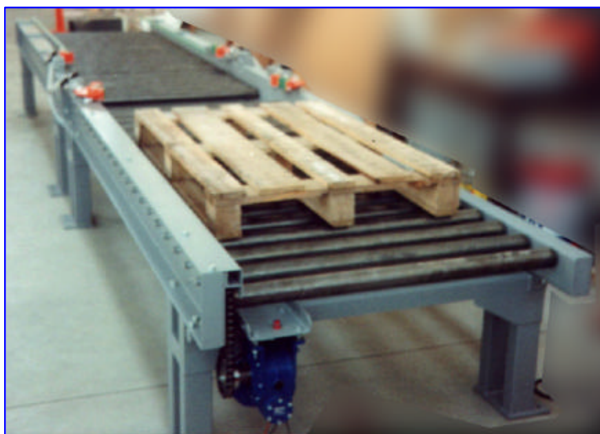
Photo 3.3 – Transporteur à rouleaux porte-pallets
